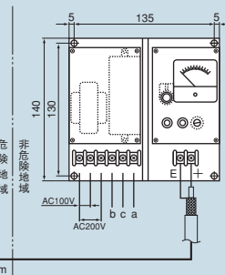
KRE6000形
