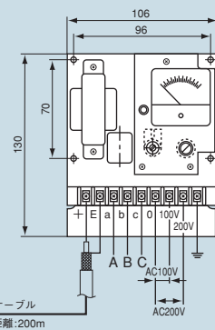
KRE6200形
