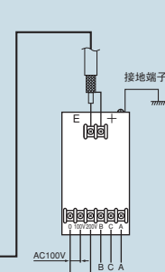
KRE6200形
