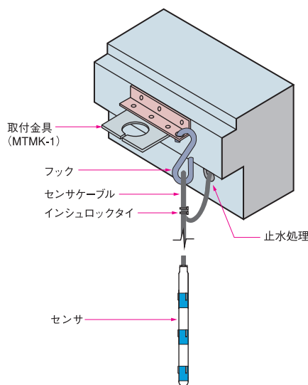
推奨センサ設置例
