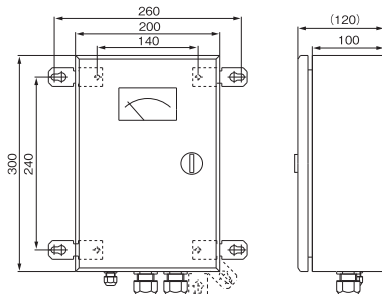
●PL4300 (中継箱) 外形
