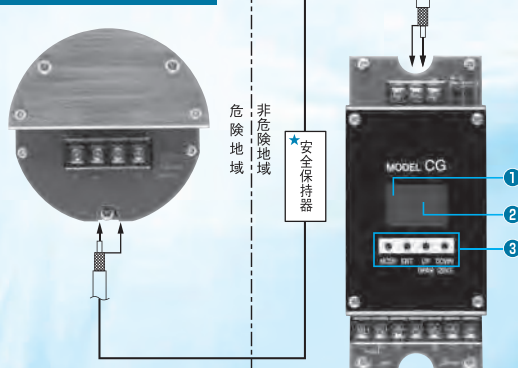
分離形(本質安全防爆)
