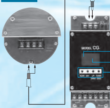
分離形
