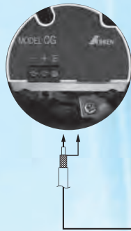
分離形(小型端子ボックス)
