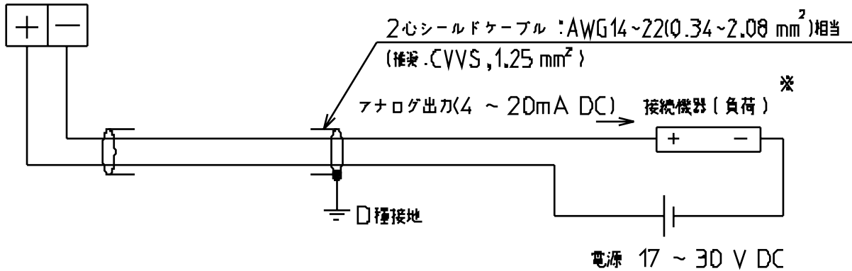
超音波式レベル計接続端子
