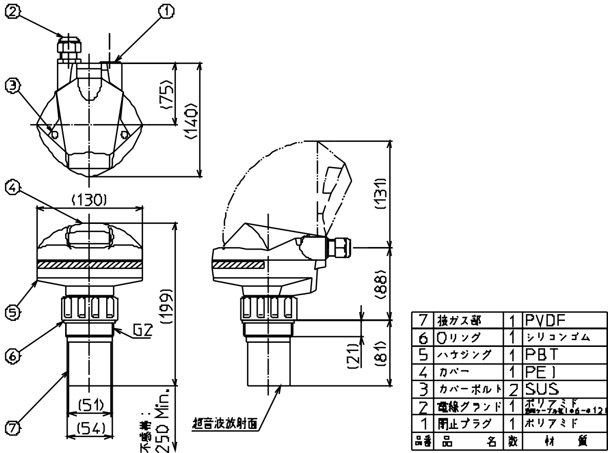
図 2 - 1 形状および寸法
