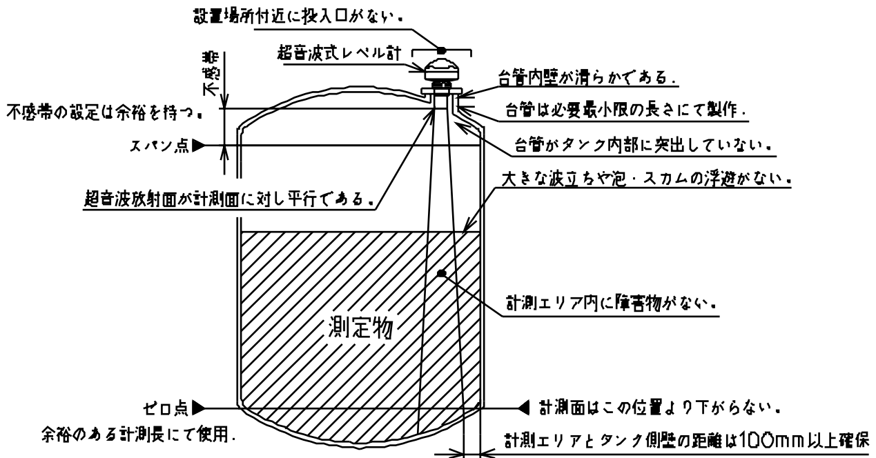
図 3 - 2 据付例
