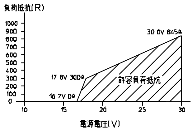
図 1 - 1 許容負荷抵抗
